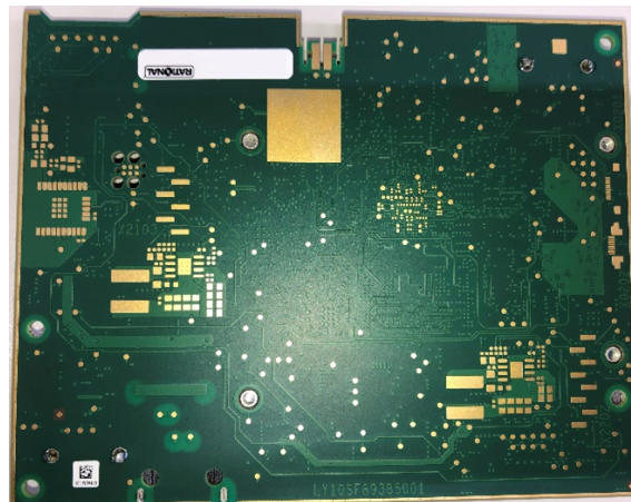
新しい代替制御ボード 背 面
